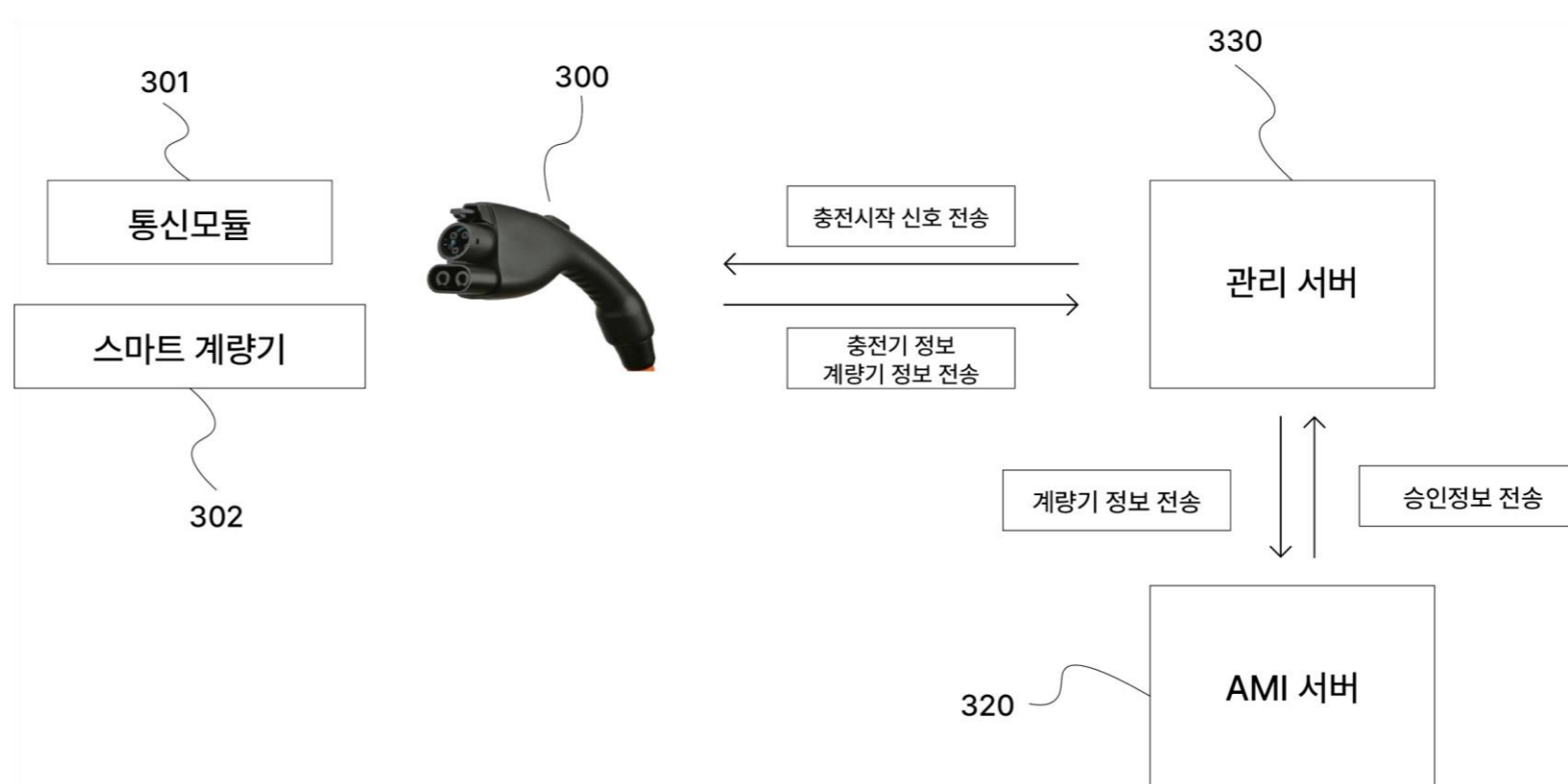
[ 특허제품 휴대용 충전기 작동 원리 ]
